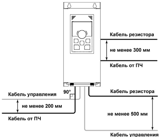
Рисунок 9 - Графическое изображение расстояний между кабелями
