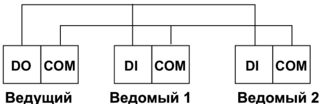
Рисунок 7 - Схема подключения управляющих клемм при параллельном подключении тормозных модулей
