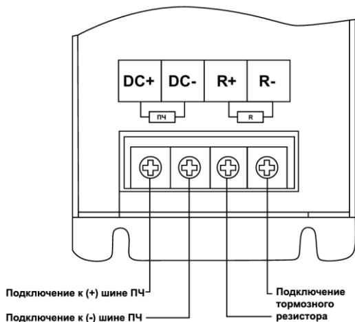
Рисунок 5 - Подключение силовых клемм одного тормозного модуля
