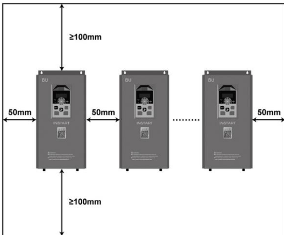
Рисунок 8 - Требуемые расстояния при монтаже тормозного модуля
