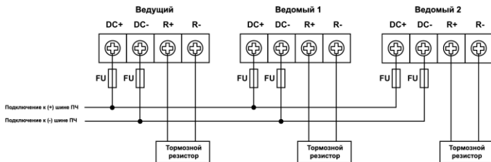
Рисунок 6 - Схема параллельного включения тормозных модулей
