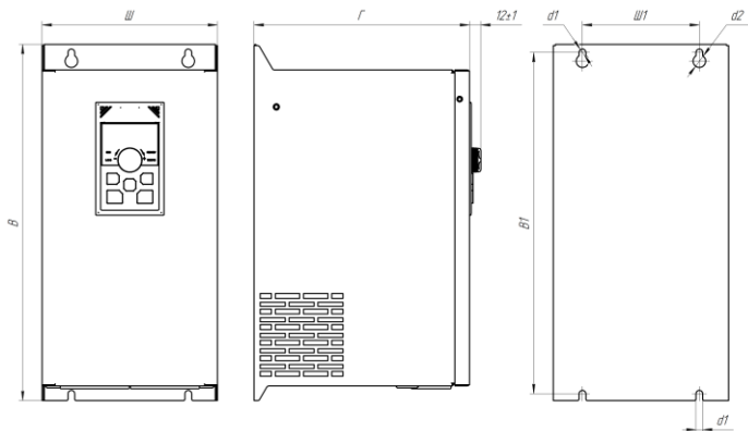
Рисунок 3 - Установочные и габаритные размеры тормозного модуля BU, типоразмер 3
