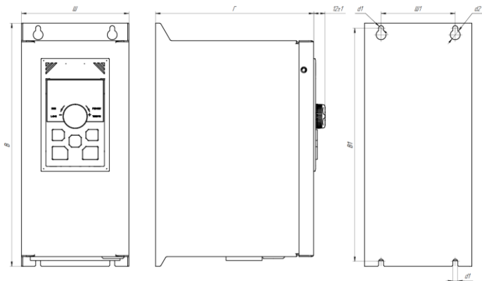
Рисунок 1 - Установочные и габаритные размеры тормозного модуля BU, типоразмер 1
