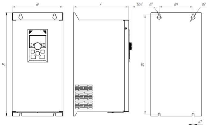
Рисунок 2 - Установочные и габаритные размеры тормозного модуля BU, типоразмер 2
